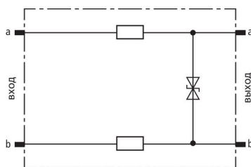
Принципиальная схема DRL RD 5
